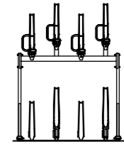
Enkelzijdig vooraanzicht 37,5 158
