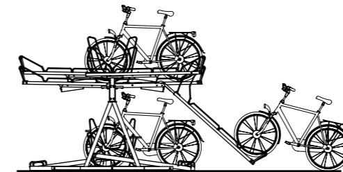
Dubbelzijdig zijaanzicht 289 96
