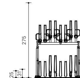
Dubbelzijdig vooraanzicht 275 37,5 165
