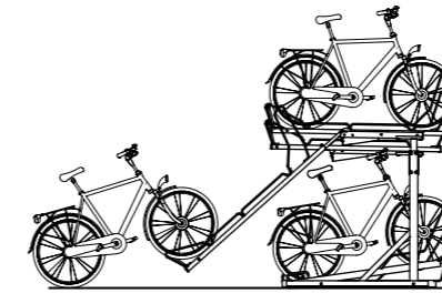
Enkelzijdig zijaanzicht 96 190
